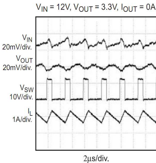
空载时波形
